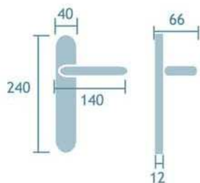
Manilla con placa Ref. 1130/SF/26D Mitos 1jgo.
