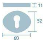
Bocallave Yale línea Monte Carlo Ref: M25KS
