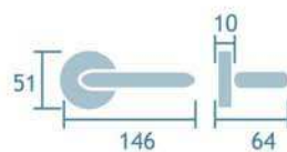
Manilla con roseta Mitos Ref. 1131/SB/26D Mitos 1jgo.
